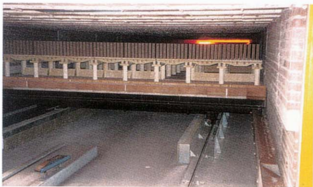
Blick in den Tunnelofen und auf die Radkühlung für die TOW – bei geöffnetem Ofenausfahrttor View into the tunnel kiln showing the wheel cooling for the tunnel kiln cars – the kiln exit door is open
