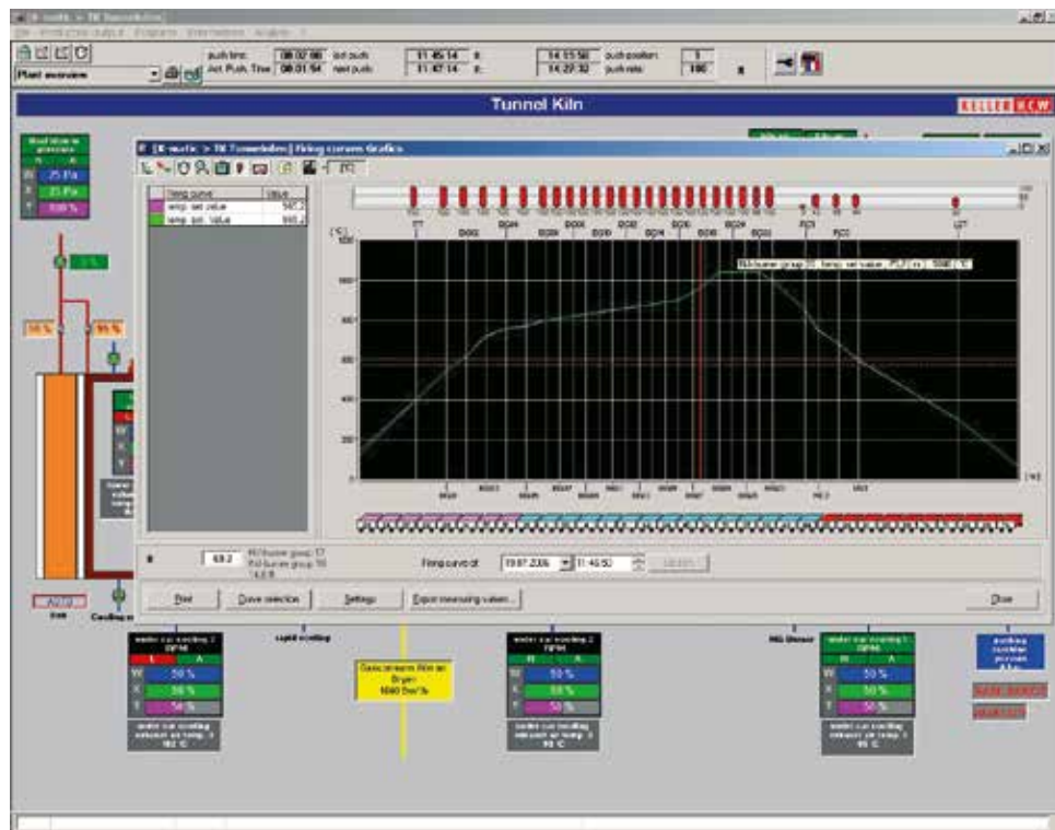
Brenn-/Trockenkurvendarstellung mit aktueller Wagenstandsanzeige Presentation of firing curve/drying curve with current car position
