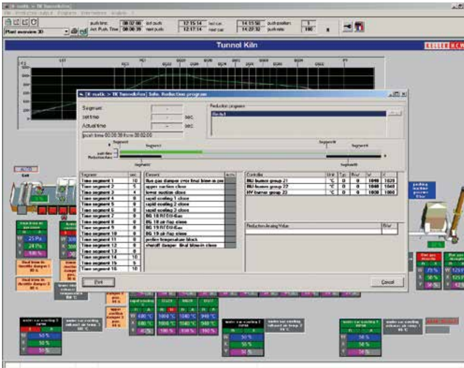
Informationen über die Reduktionssteuerung Information on reduction control
