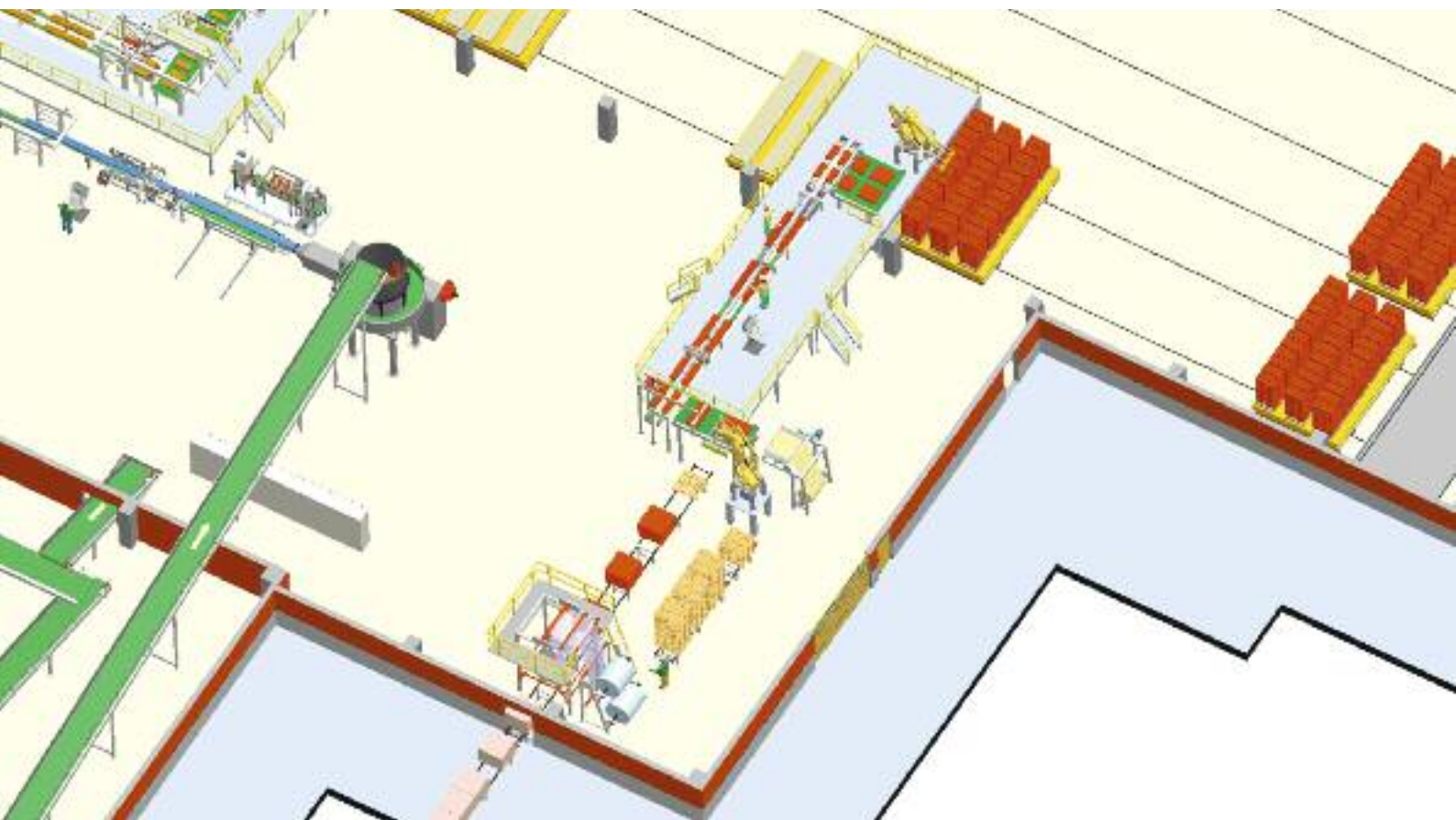
Entlade- und Verpackungsanlage Участок разгрузки и упаковки
