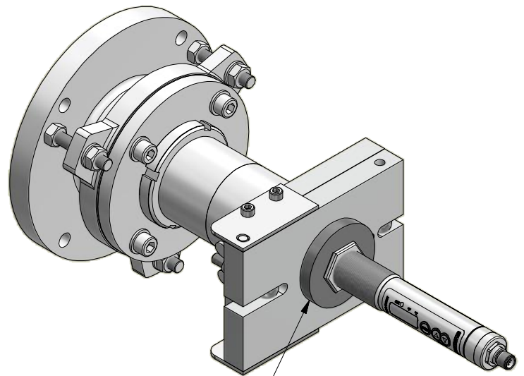
Montagebeispiel Mounting example
