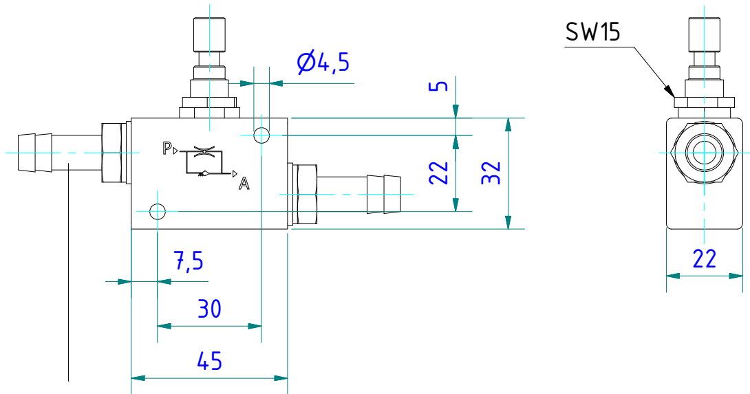
Schlauchtülle G1/4" für Schlauch mit lichter Weite 8 bis 9 mm Hose nozzle G1/4" for hose with inner width 8 to 9 mm
