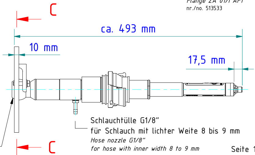
Kugelflansch ball flange
